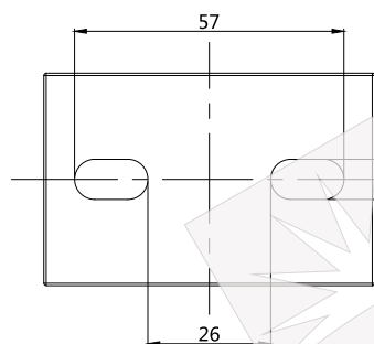
安装支架孔位尺寸图
