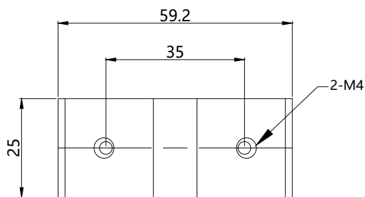
安装支架孔位尺寸图
