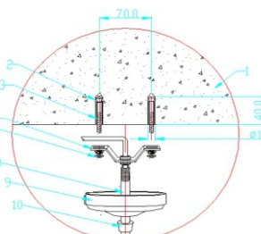
预埋膨胀大螺帽
