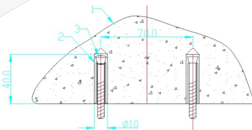
水泥天花板安装孔打孔示意图
