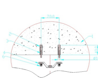
预埋膨胀大螺帽
